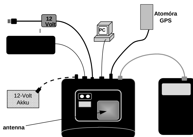
Egyesületi gyűjtőantenna csatlakozásának ábrája
